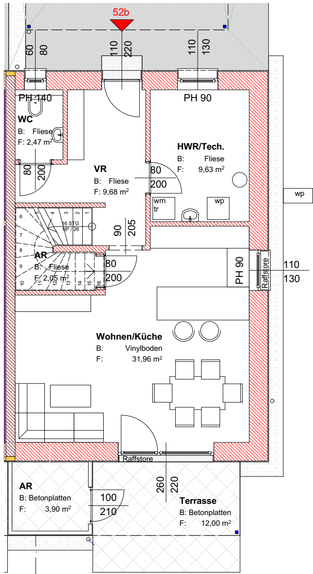
0. Erdgeschoss 1:100
