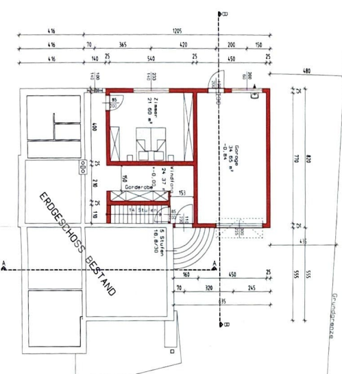
ERDGESCHOSS
