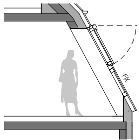
SCHNITT B
