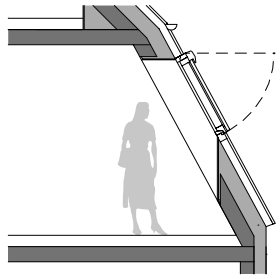
SCHNITT A
