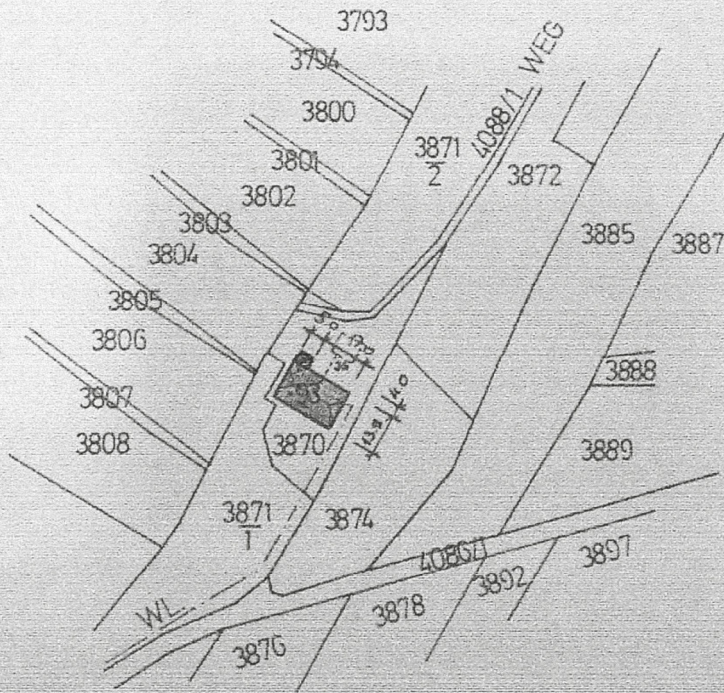
LAGEPLAN M 1:2000
