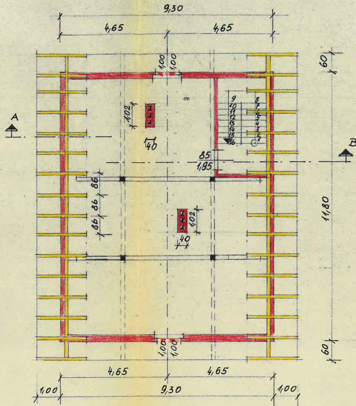
Dachgeschoß
