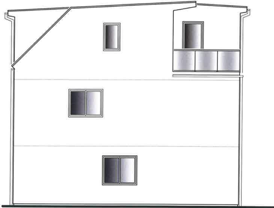
SÜDWEST ANSICHT TOP 1
