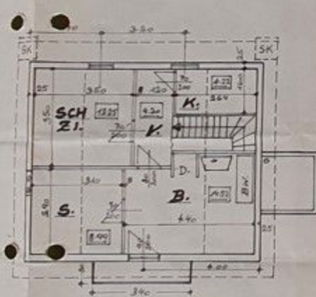
DACHGESCHOSS
