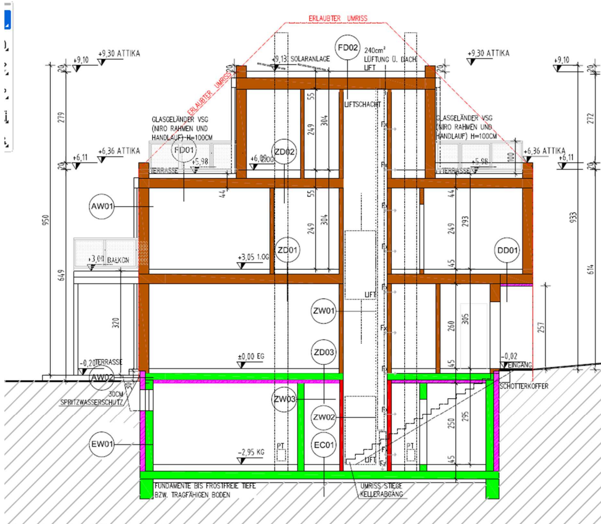
SCHNITT A-A
