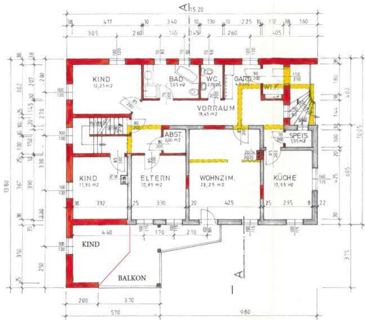
ERDGESCHOSS
