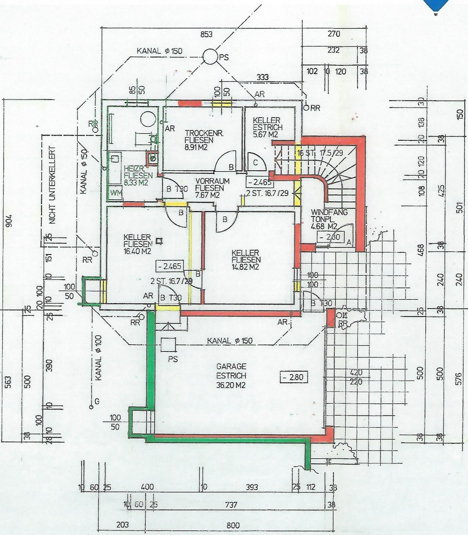
KELLERGESCHOSS
