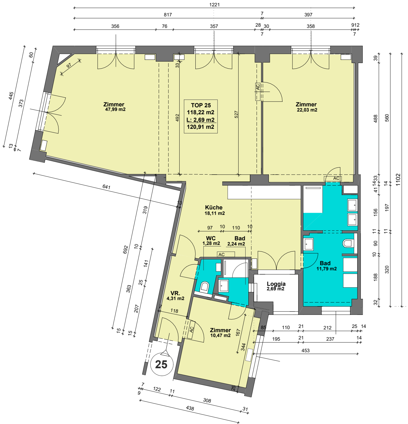
HERRENGASSE 6-8, STIEGE 2, 6. STOCK, TOP 25, 18.06.2024 M 1:100
