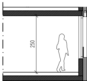
SCHNITT B2
