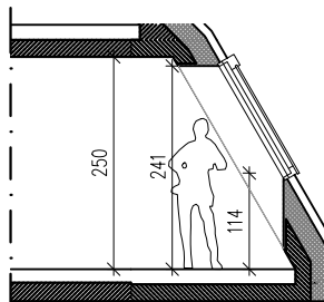
SCHNITT B3
