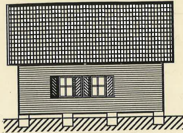
Ostansicht
