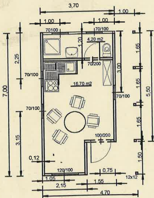
Erdgeschoß
