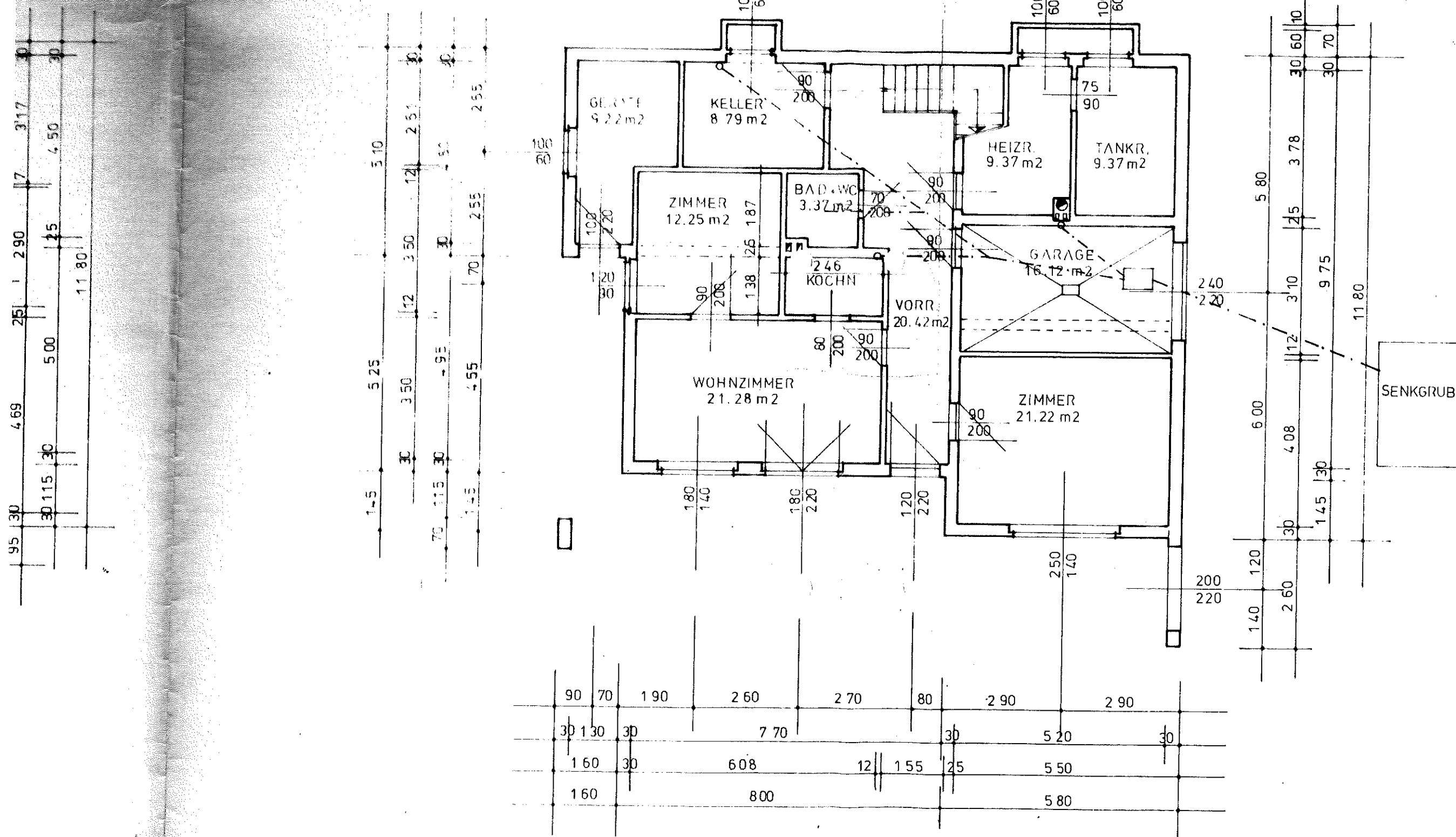
GRUNDRISS KELLERGECHOSS
