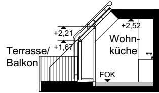
Querschnitt 2 M:1:150
