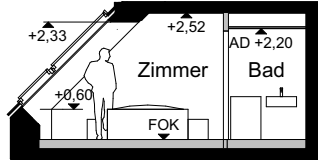
Querschnitt 1 M:1:150
