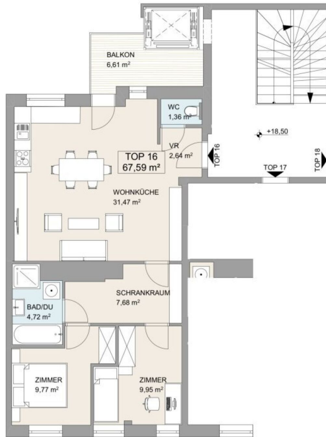
2. DACHGESCHOSS
