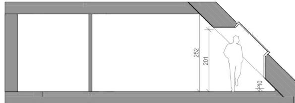
Schnitt 1-1
