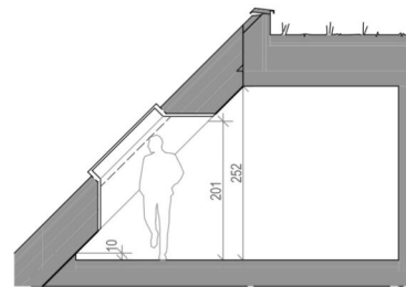
Schnitt 1-1
