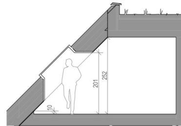
Schnitt 1-1
