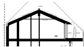
SCHNITT 3.OG M=1:200
