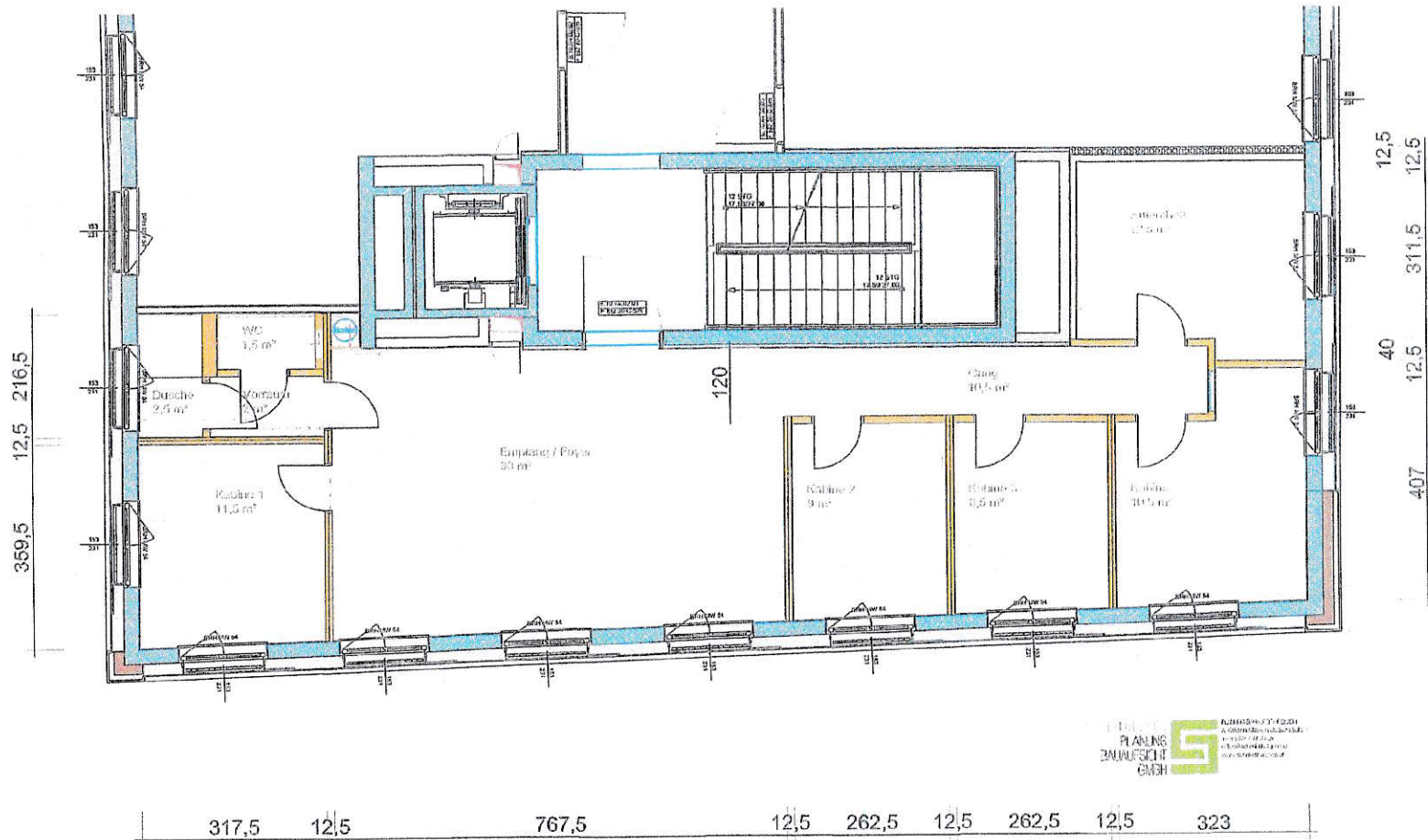
Beilage /B Planskizze mit Zwischenwänden und WC-Anlage
