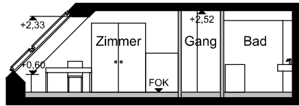
Querschnitt M:1:150
