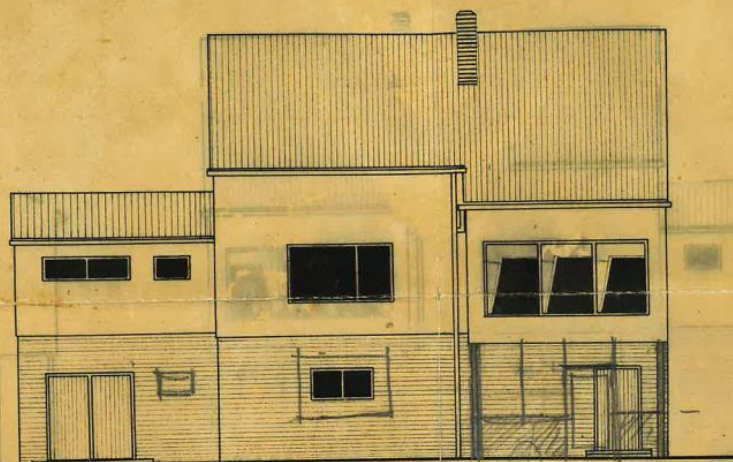
Westansicht
