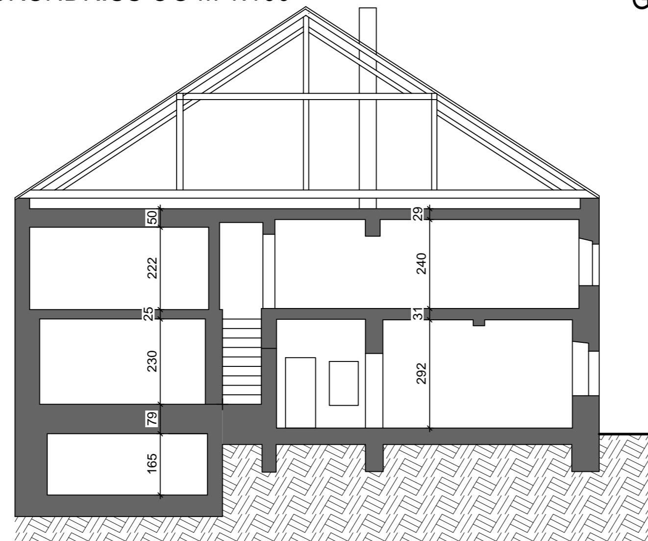
SCHNITT M 1:100
