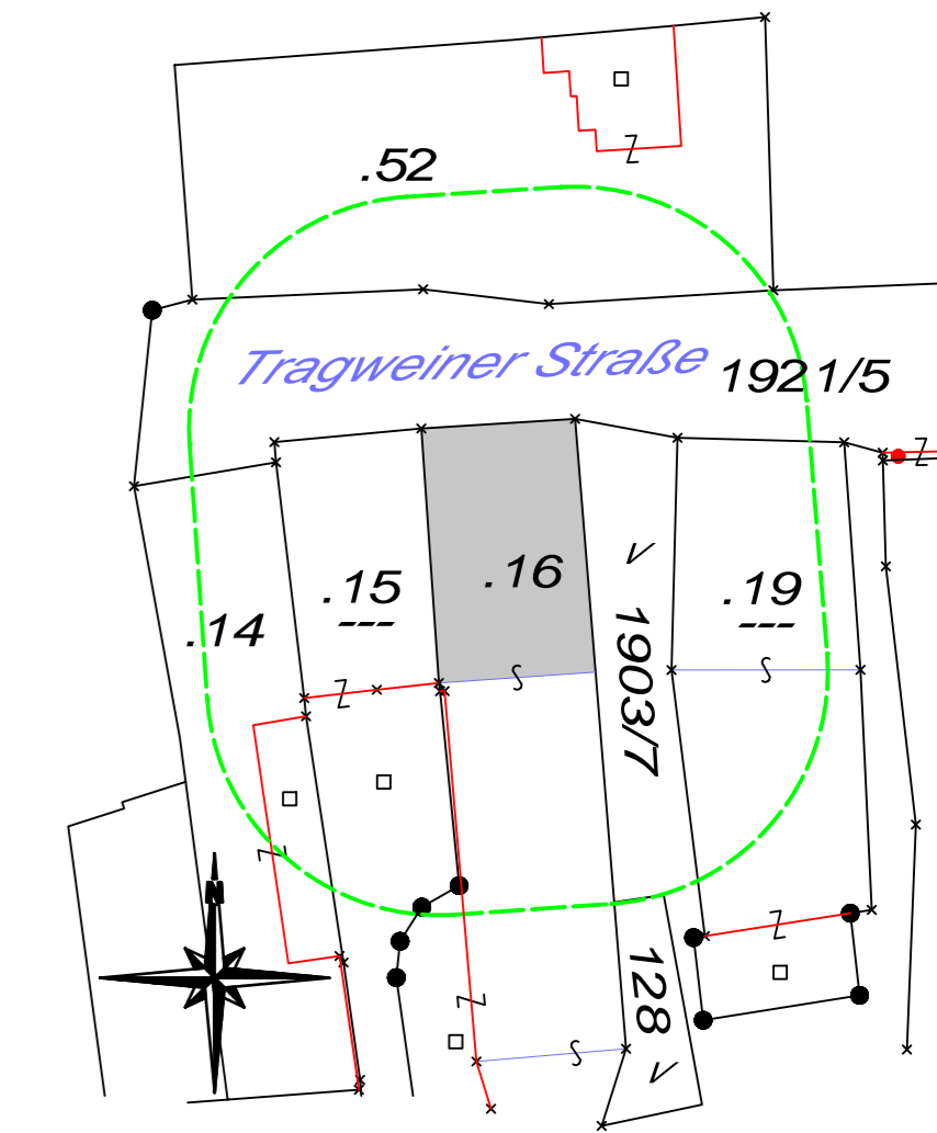
LAGEPLAN M 1:500
