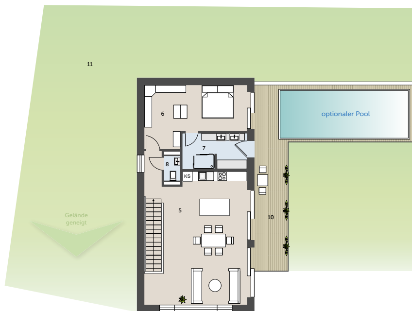
2. OBERGESCHOSS
