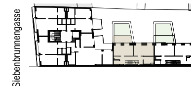
Grundriss 1. Obergeschoss
