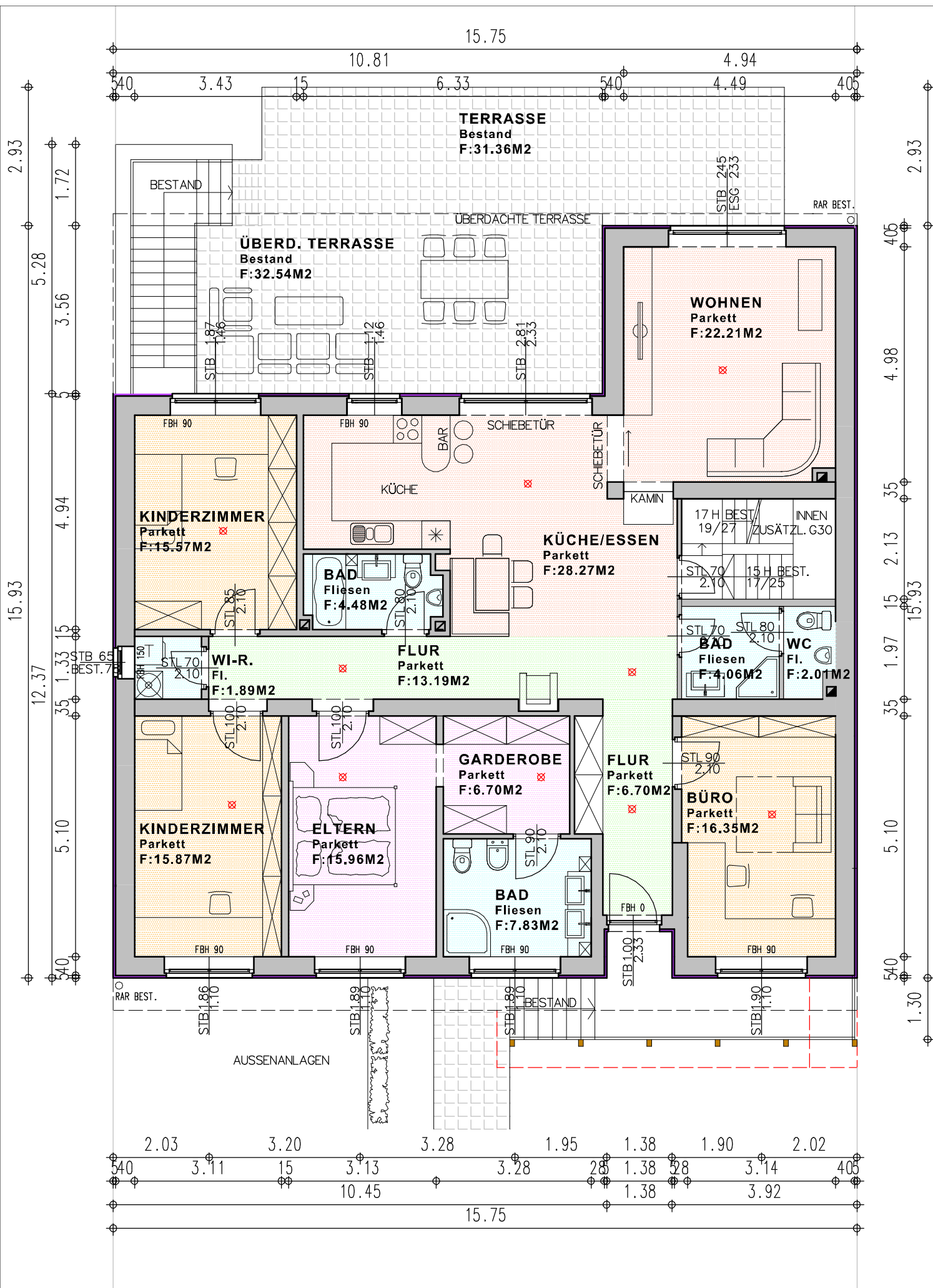
GRUNDRISS ERDGESCHOSS
