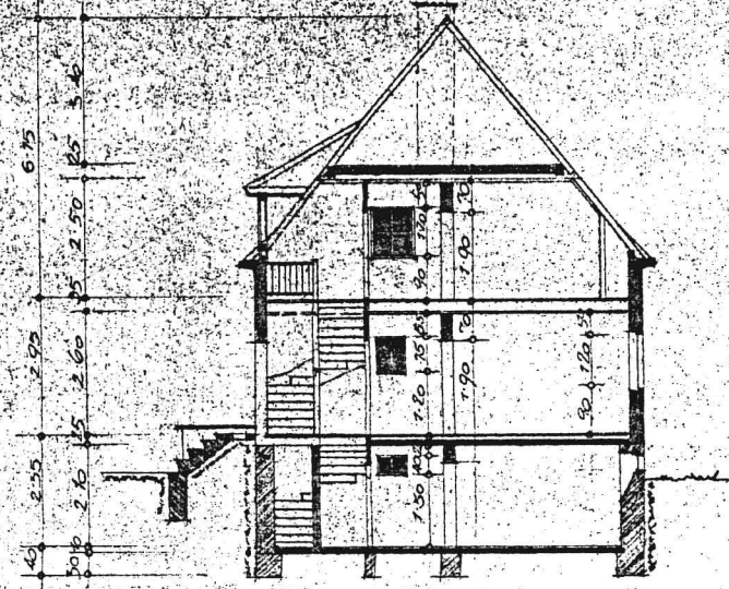
QUERSCHNITT
