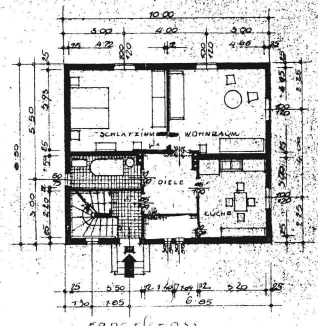
ERDGESCHOSS
