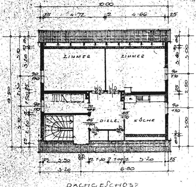
DACHGESCHOSS
