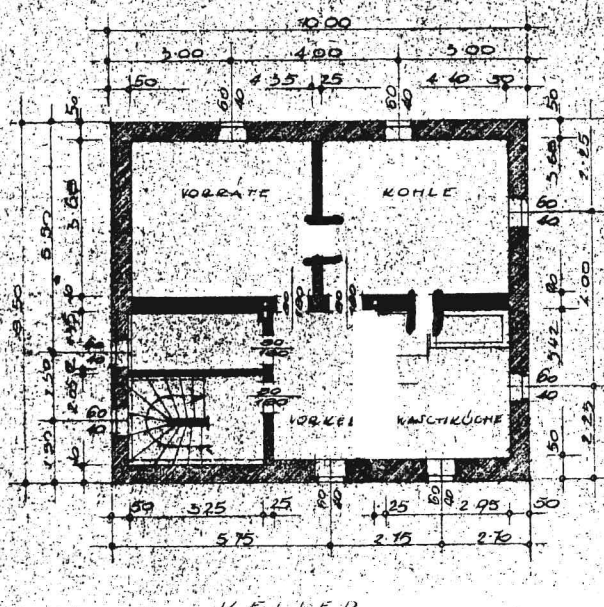
KELLER
