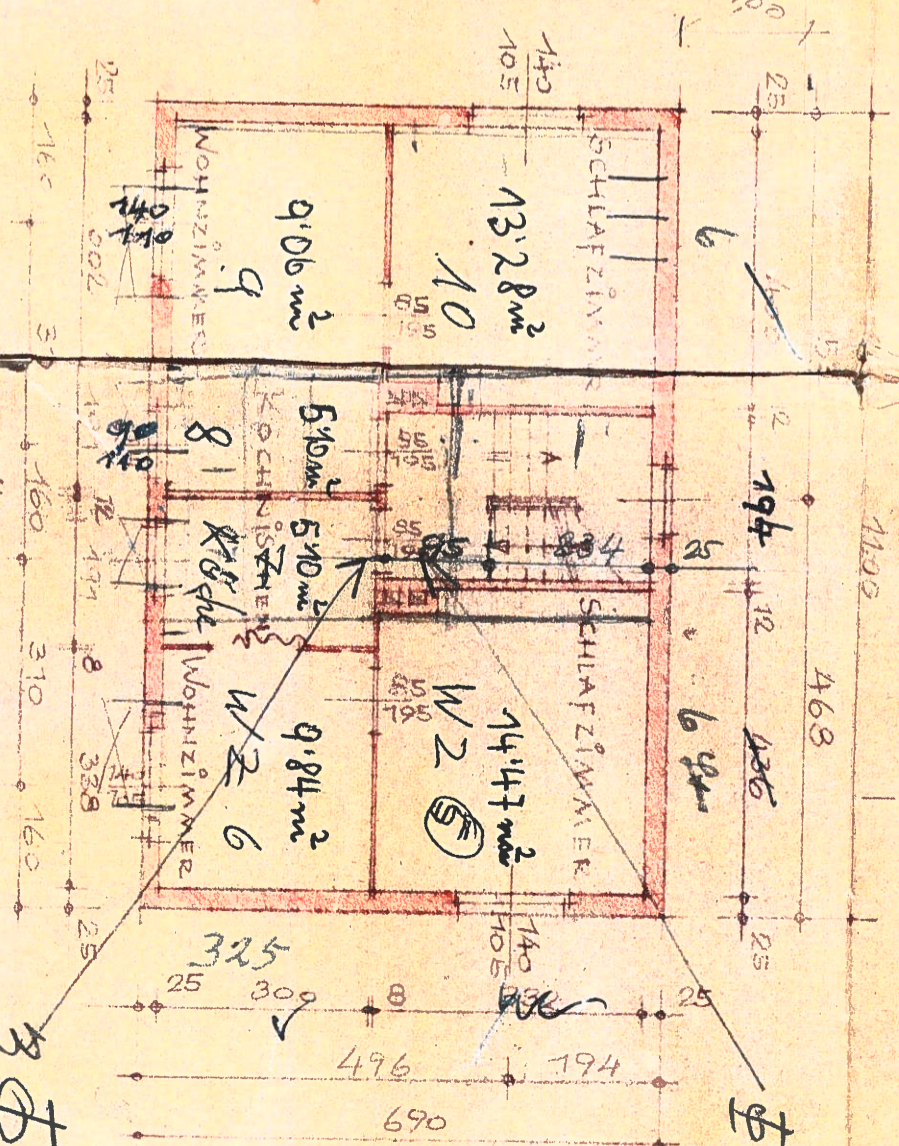
ERDGESCHOSS
