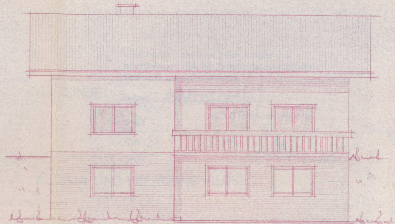
SÜD-WEST ANSICHT
