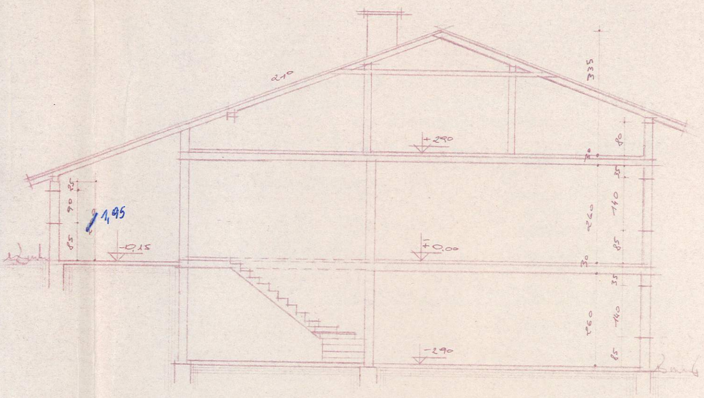
SCHNITT
