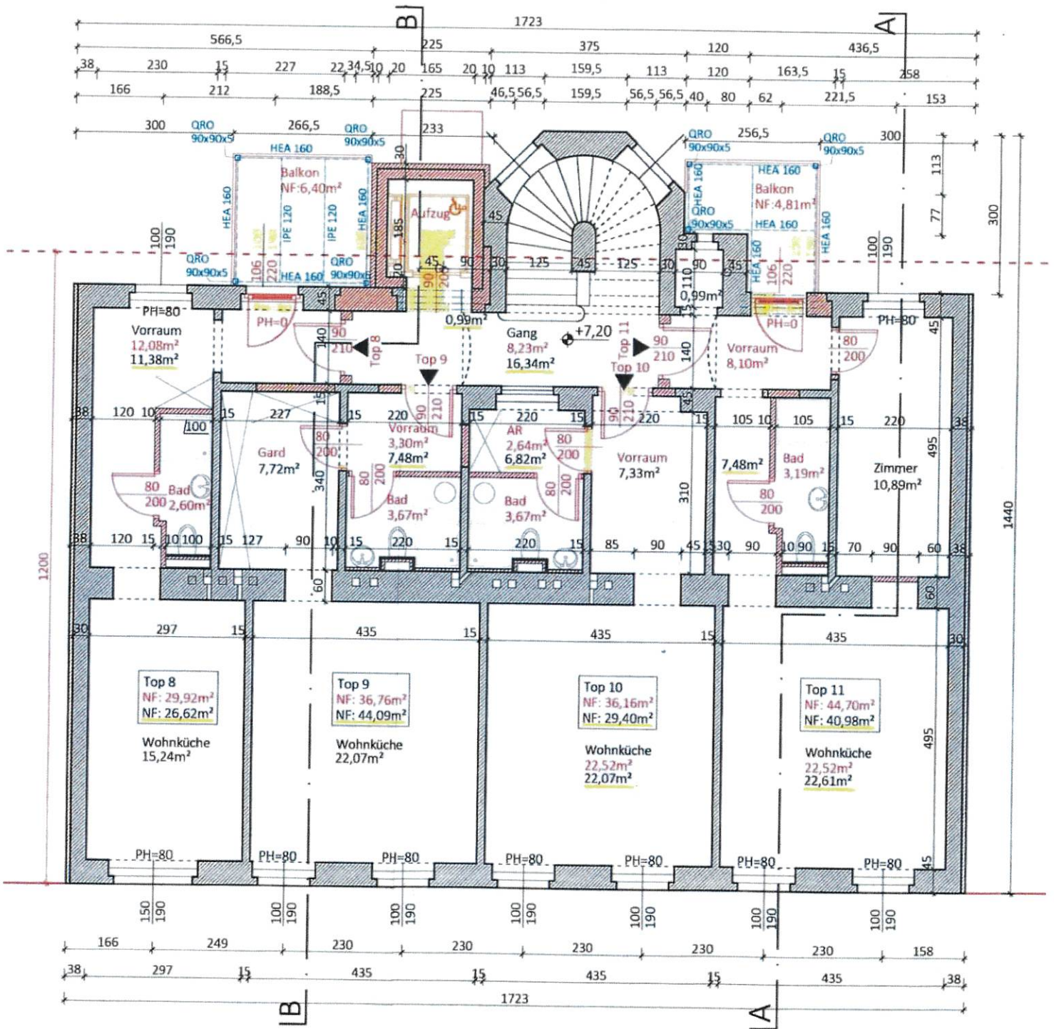
Grundriss 2.Obergeschoss
