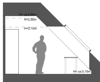
SCHNITT B
