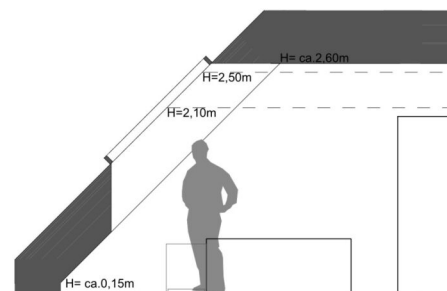
SCHNITT A
