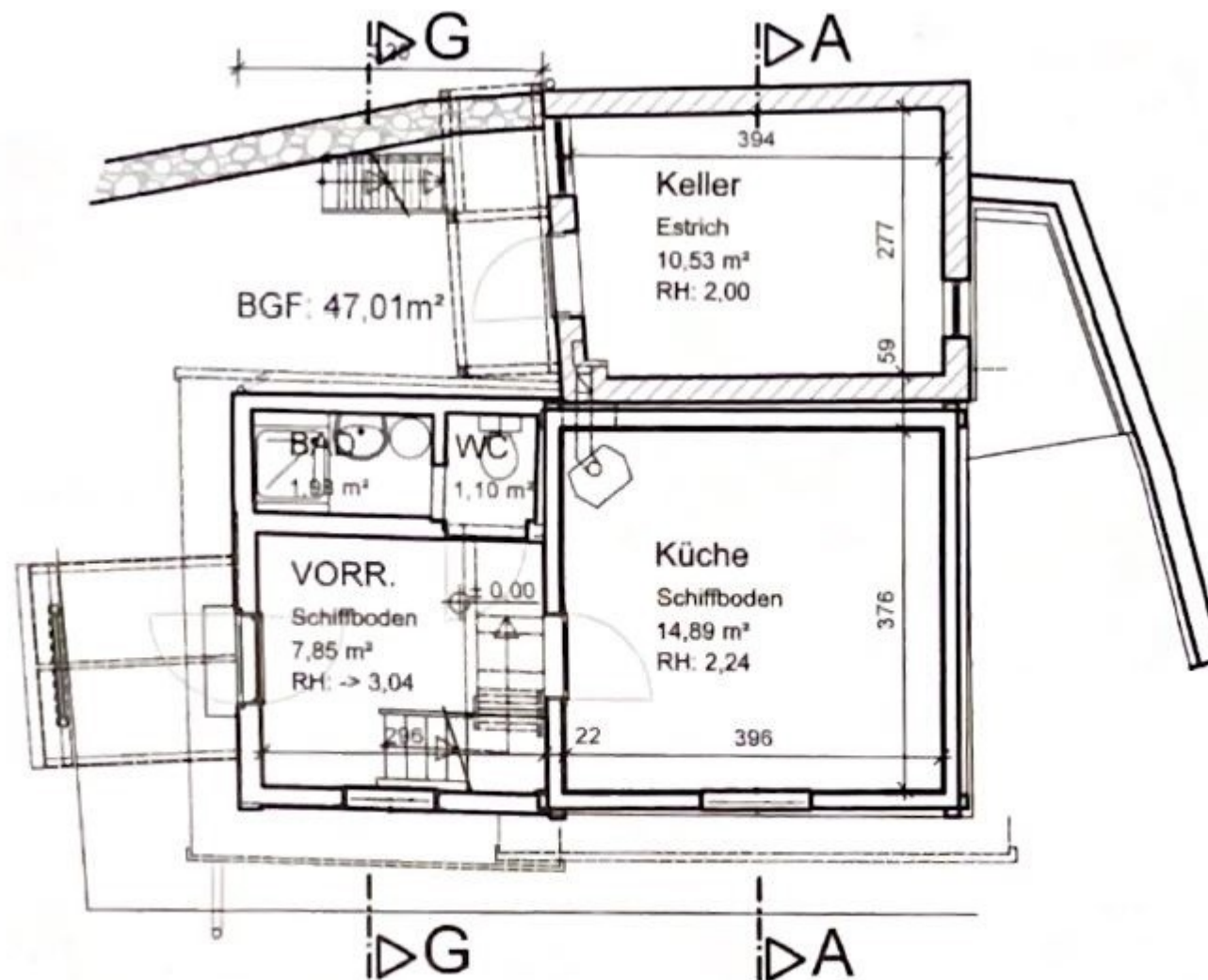
Grundriss Erdgeschoß
