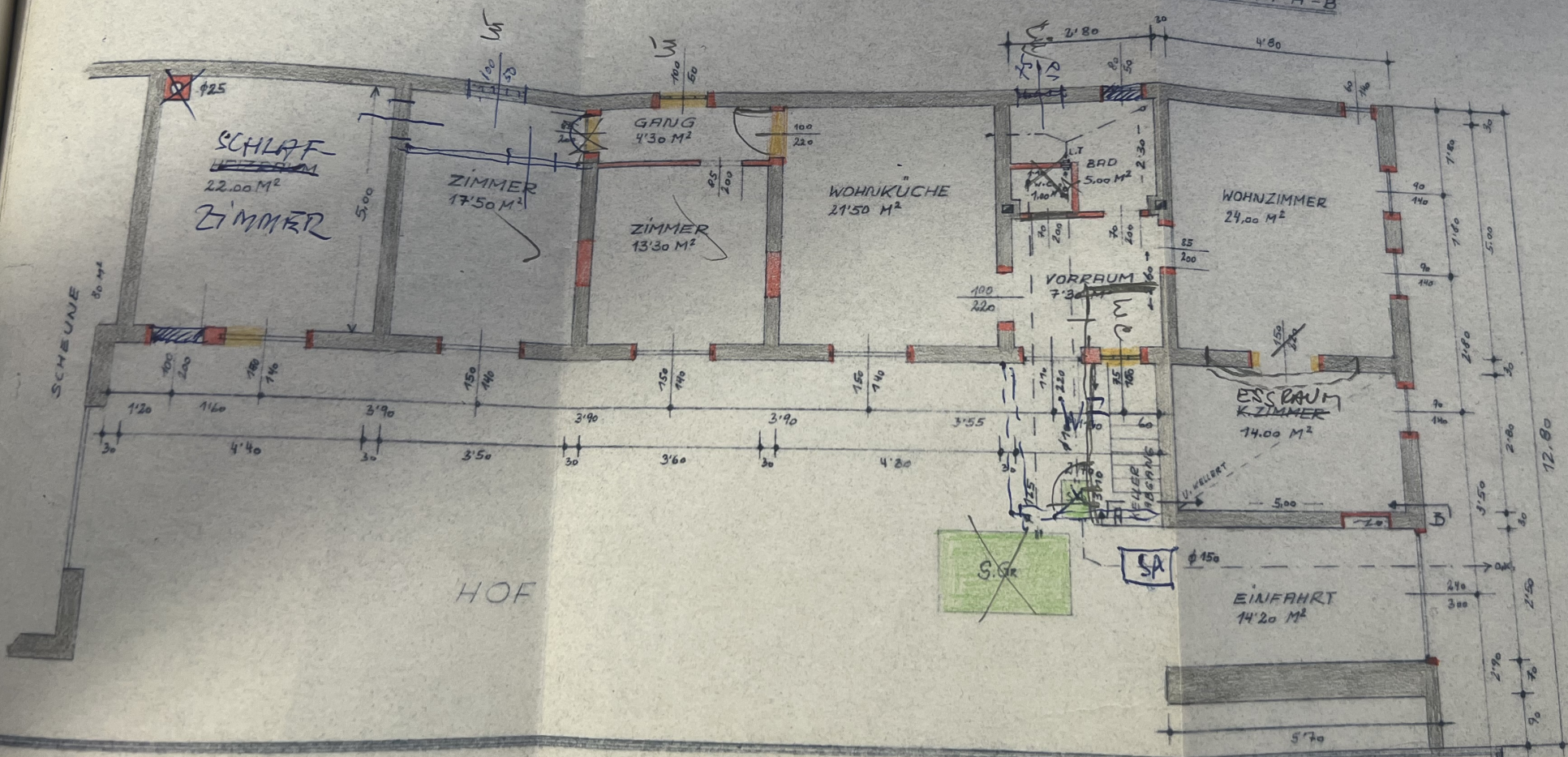
GRUNDRISS
