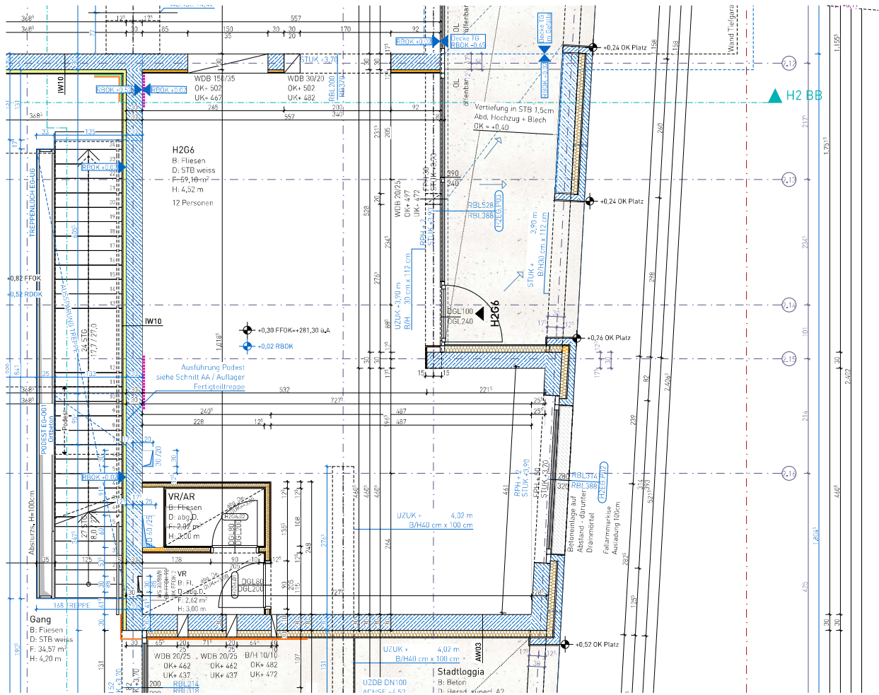
GRUNDRISS H2G6 Eisdielen M=1:50
