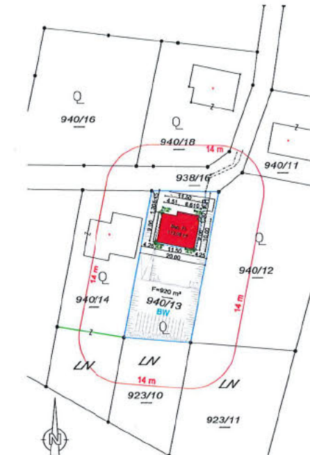
LAGEPLAN M 1:500
