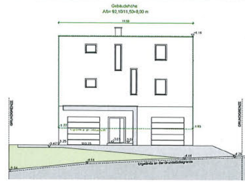
NORDANSICHT
