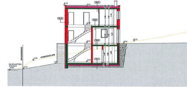
SCHNITT A-A
