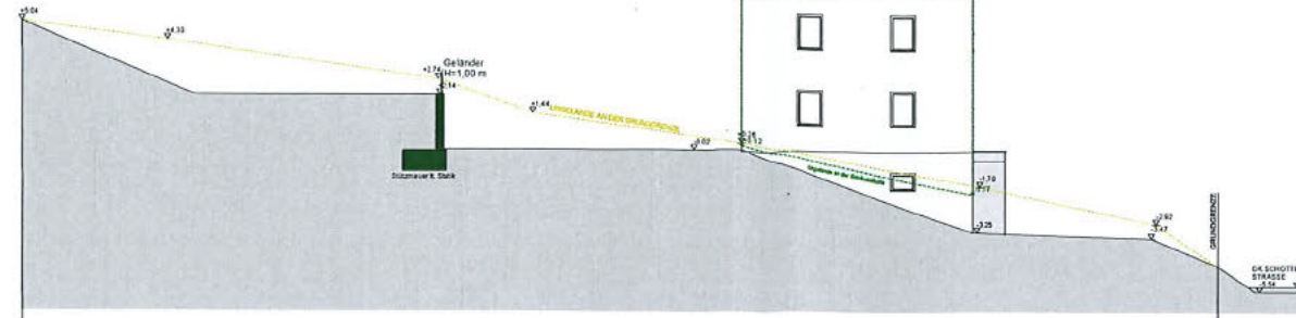
OSTANSICHT
