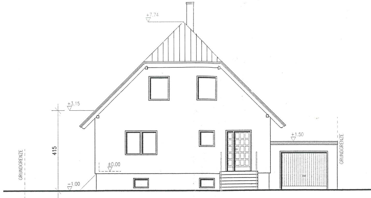
ANSICHT SUED-OST
