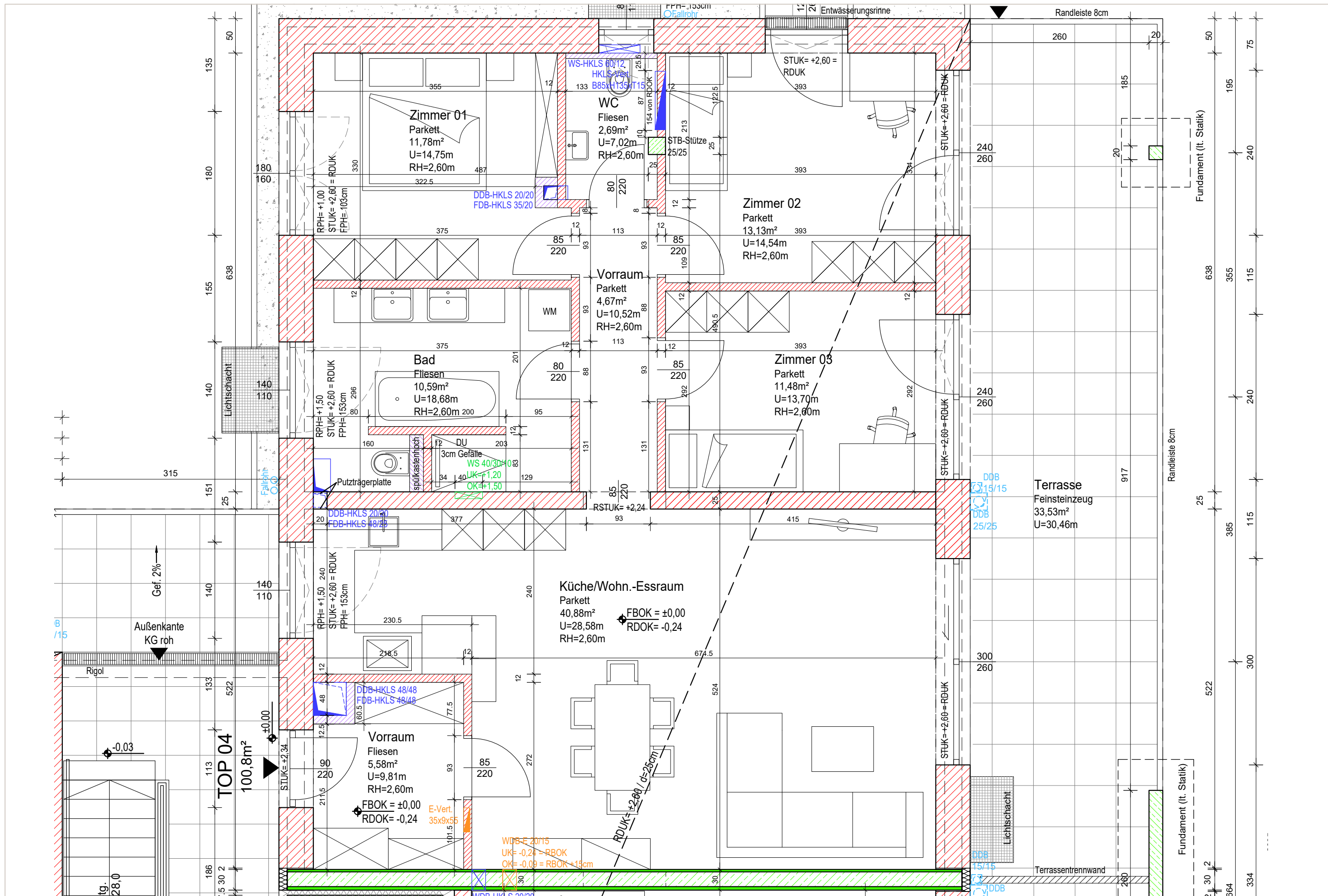
Wohnanlage Klosterkogelstraße Grundriss TOP04 1:50 20210929
