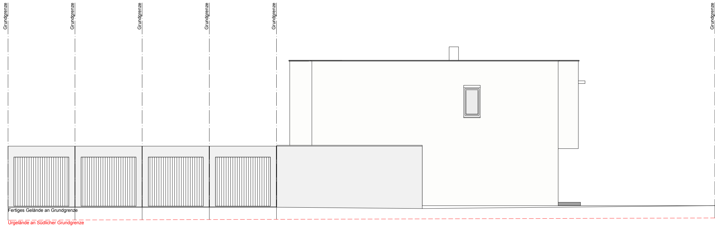
SÜD ANSICHT
