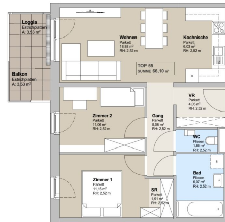
3. Obergeschoß M: 1: 100
