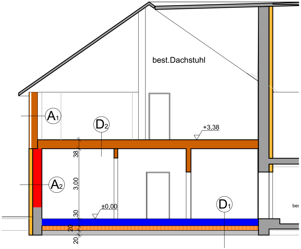
Schnitt C-C M=1:100
