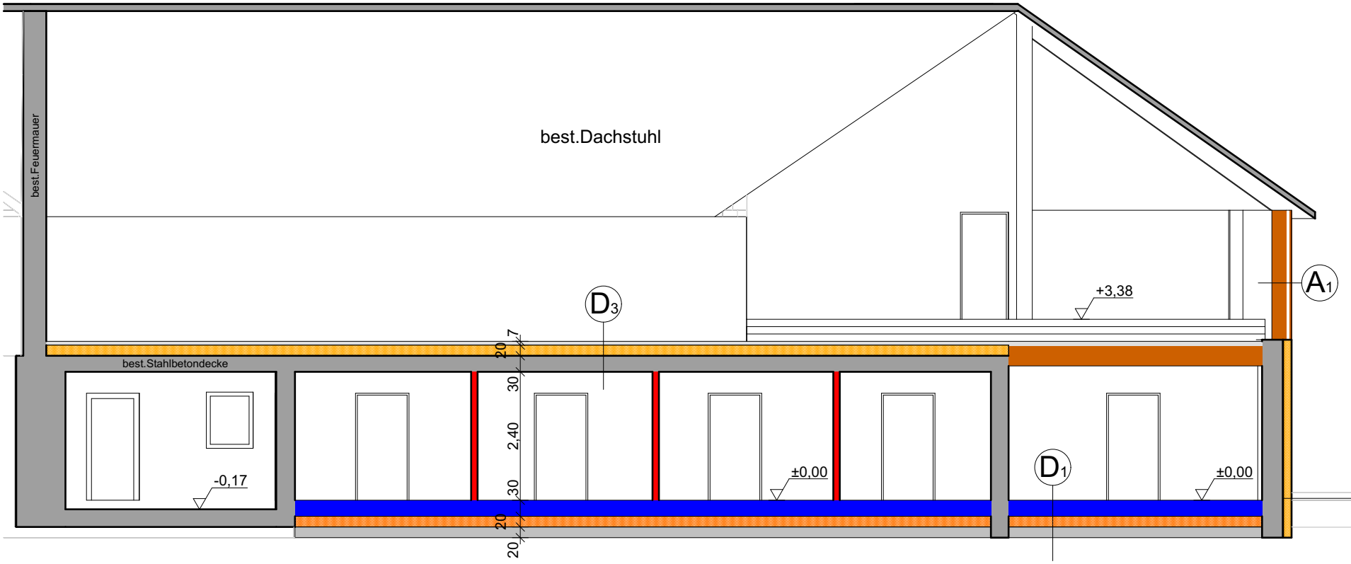
Schnitt D-D M=1:100
