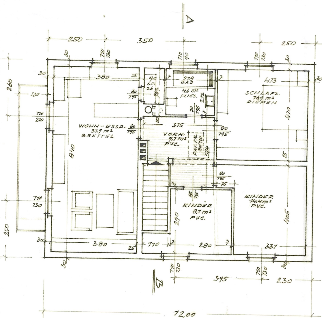
OBERGESCHOSS
