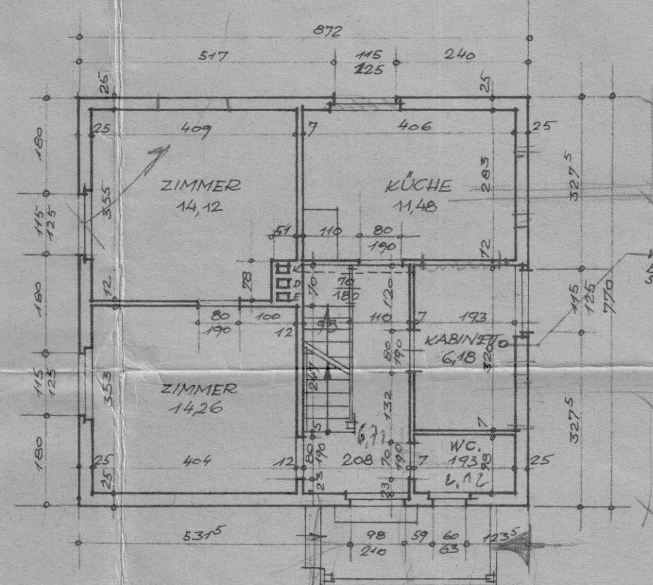
ERDGESCHOSS
