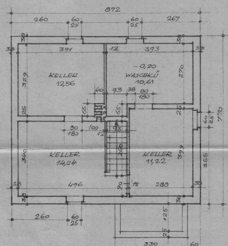
KELLER
