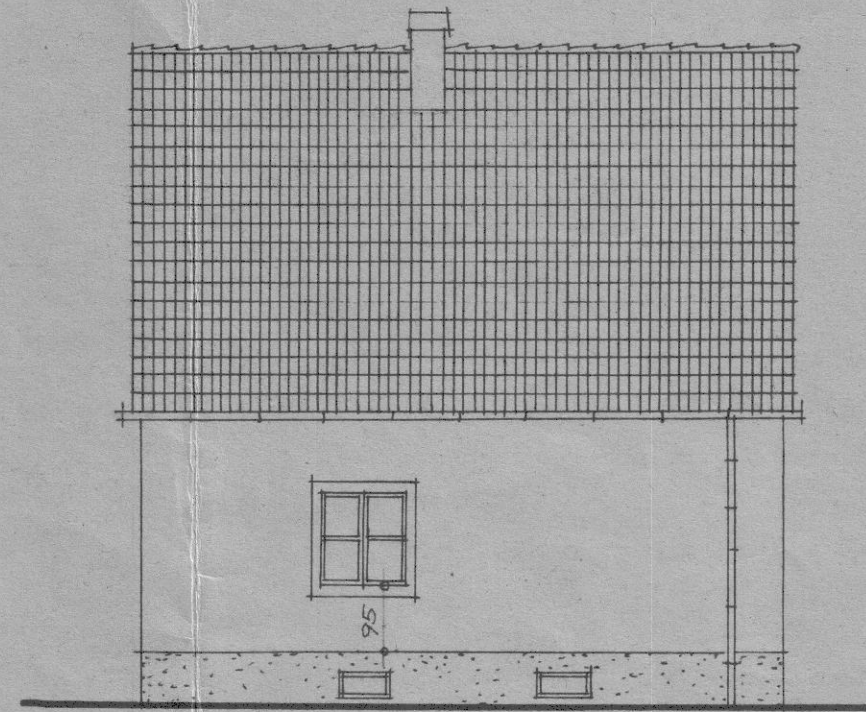
TRAUFENSEITE - WEST
