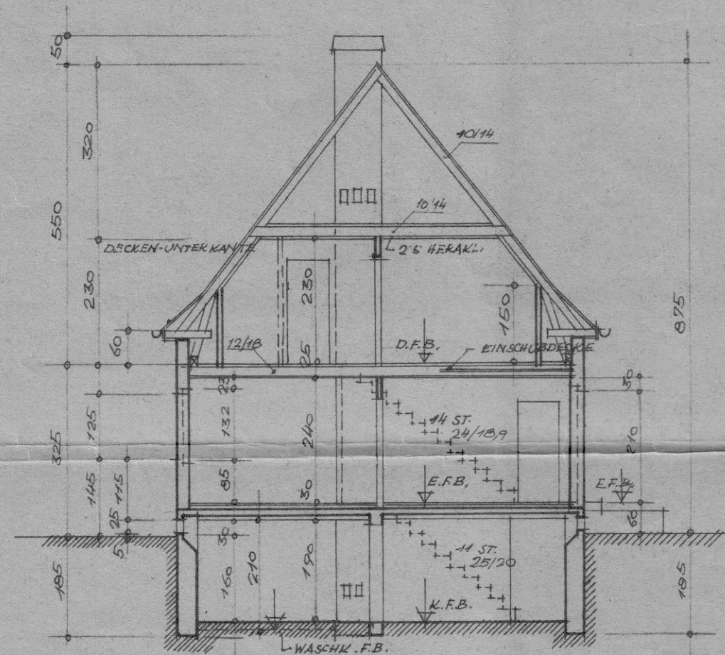
SCHNITT
