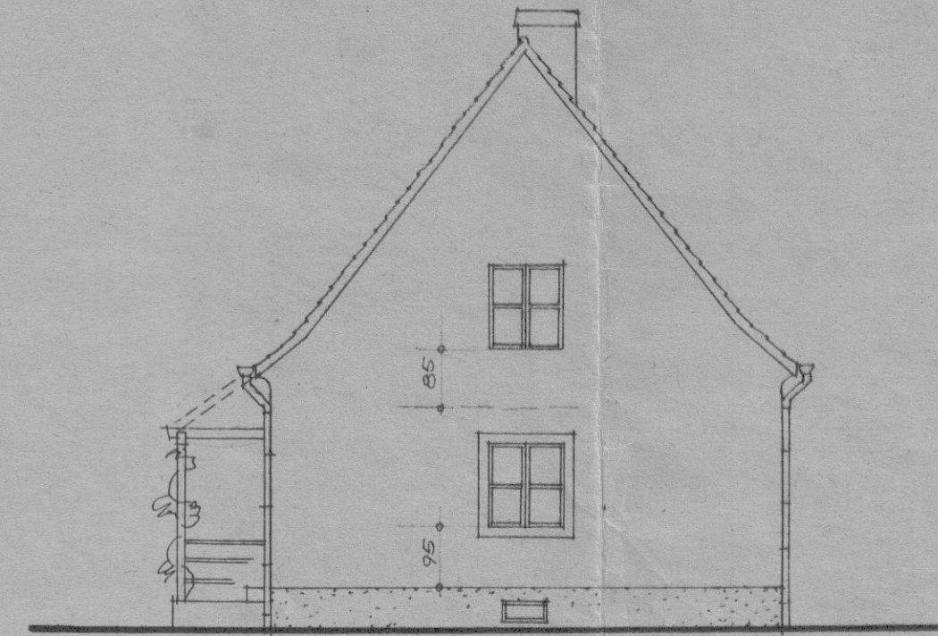
GIEBELSEITE - NORD
