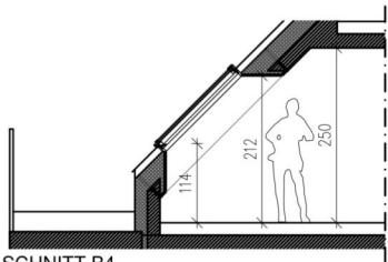
SCHNITT B4
