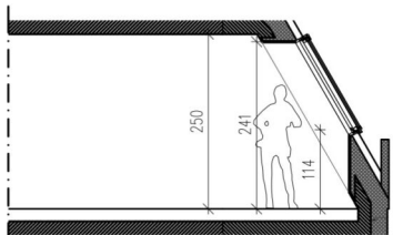
SCHNITT B3
