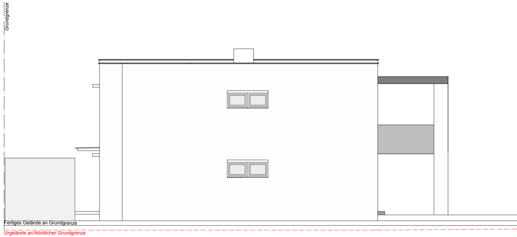
NORD ANSICHT
