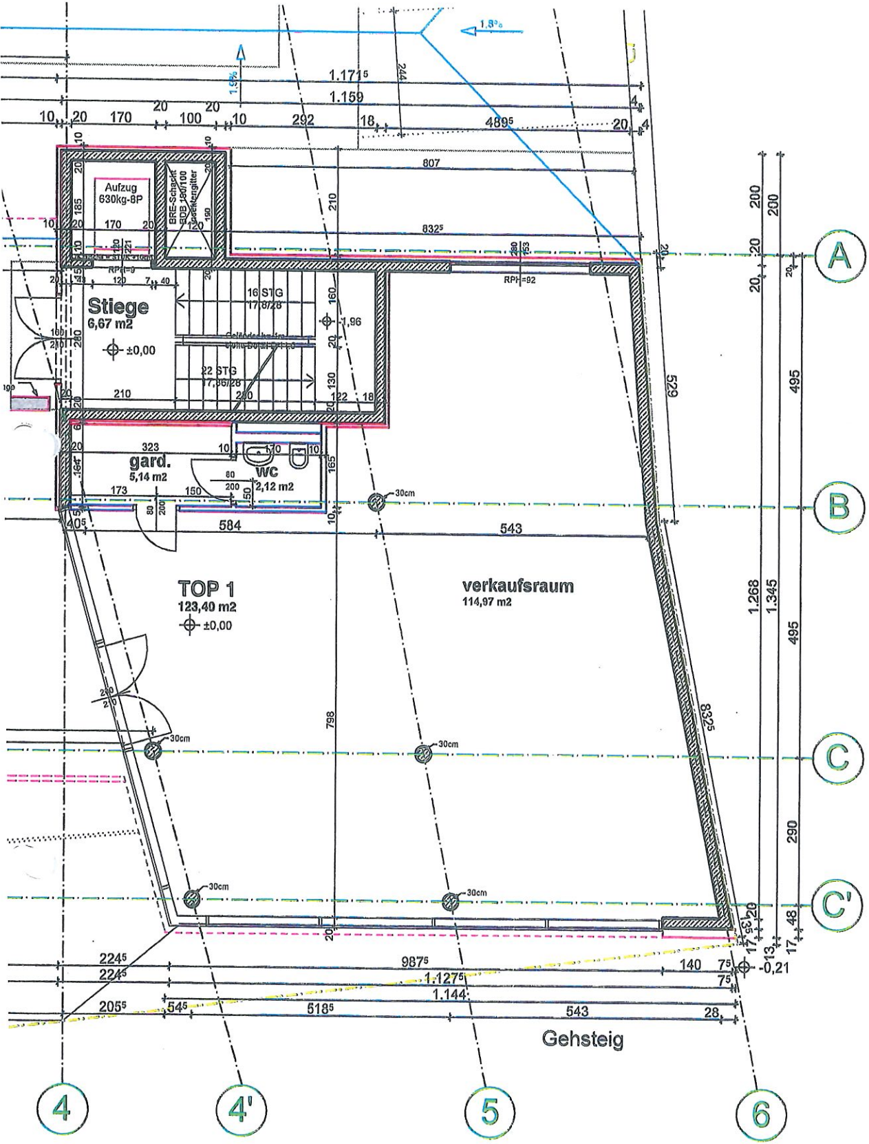
Erdgeschoss M 1:100
