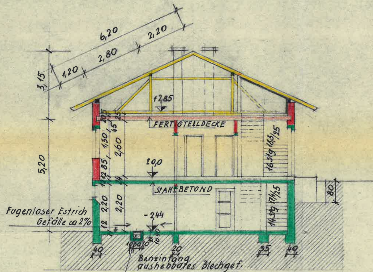
Schnitt A-B
