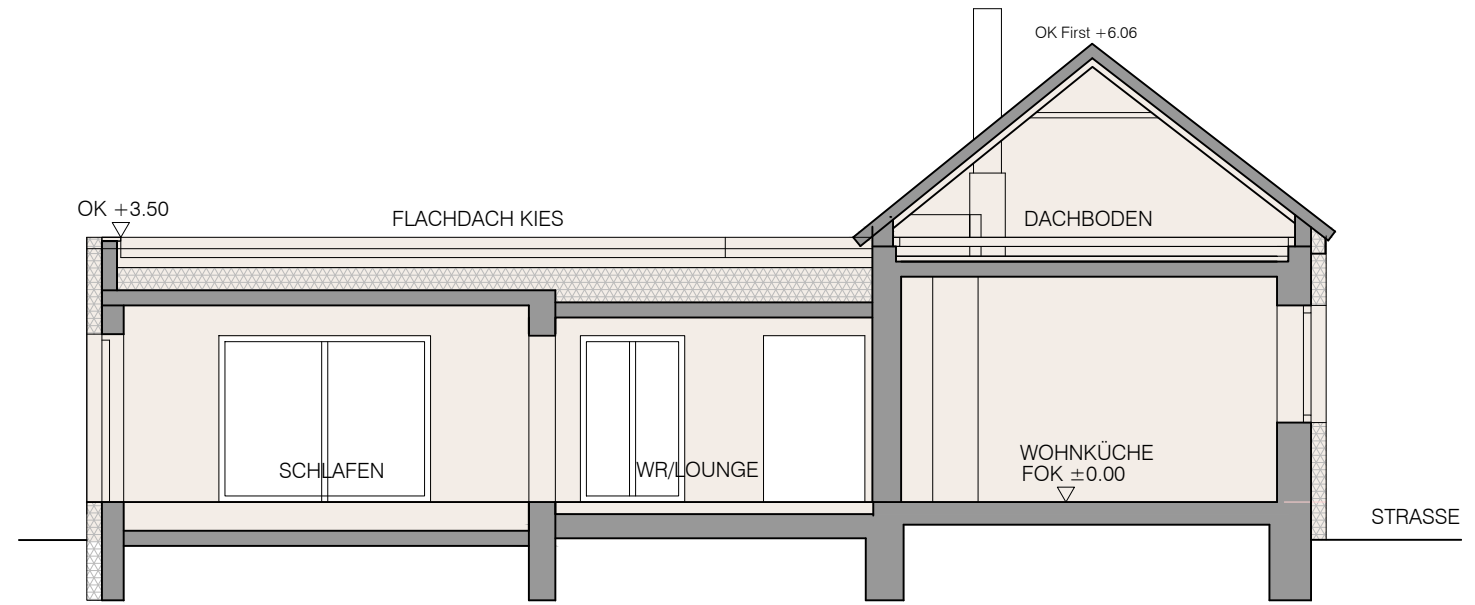
SCHNITT 2
