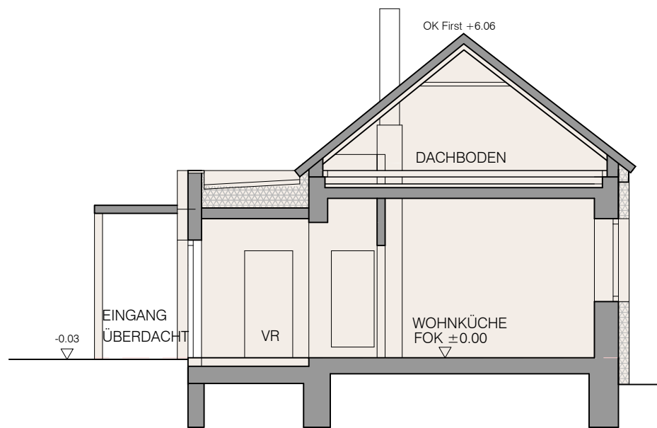
SCHNITT 1
