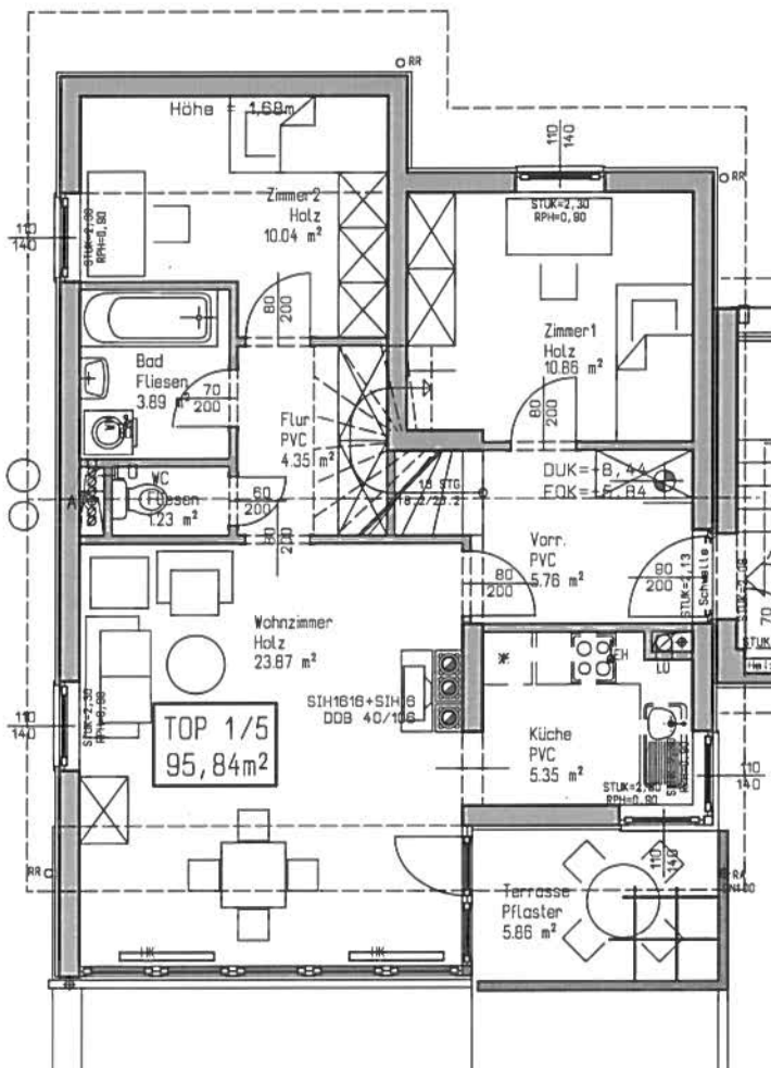
Dachgeschoss
