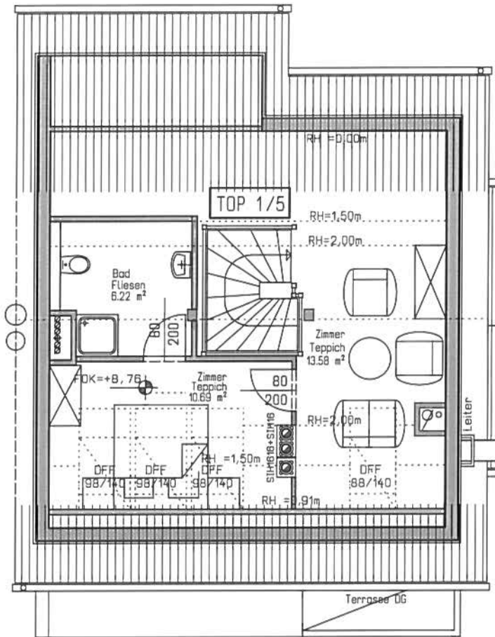
Dachboden
