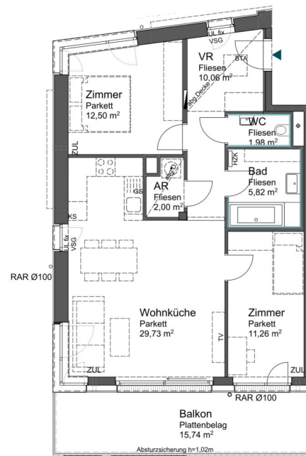
Lage Wohnung
