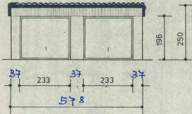
Vorderansicht:
