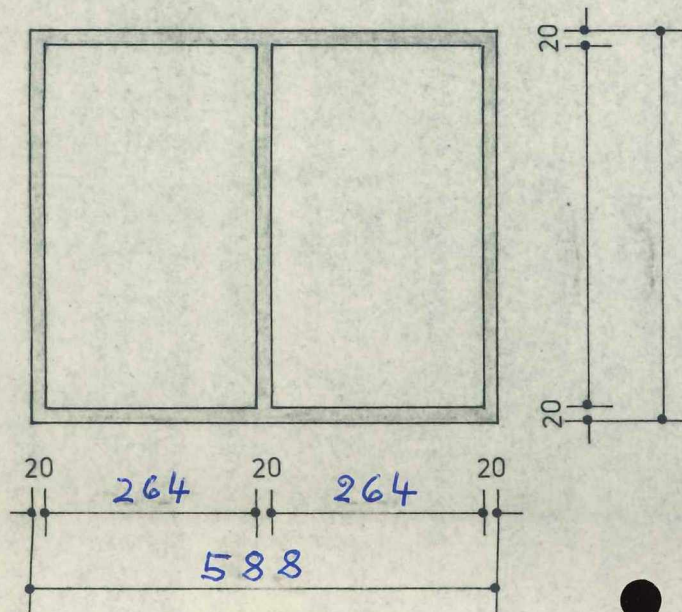
Fundament - Grundriss:
