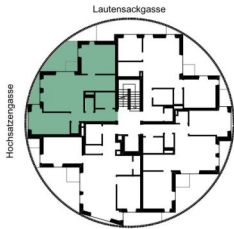
GESCHOSSPLAN
